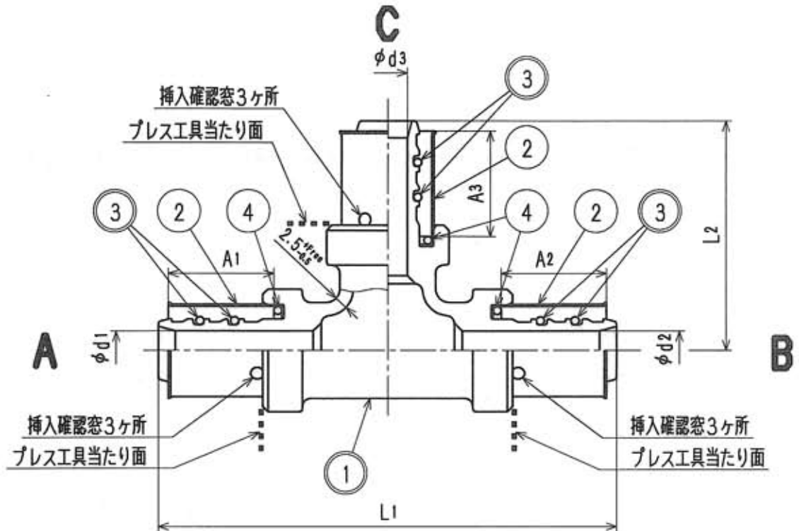
寸法表
