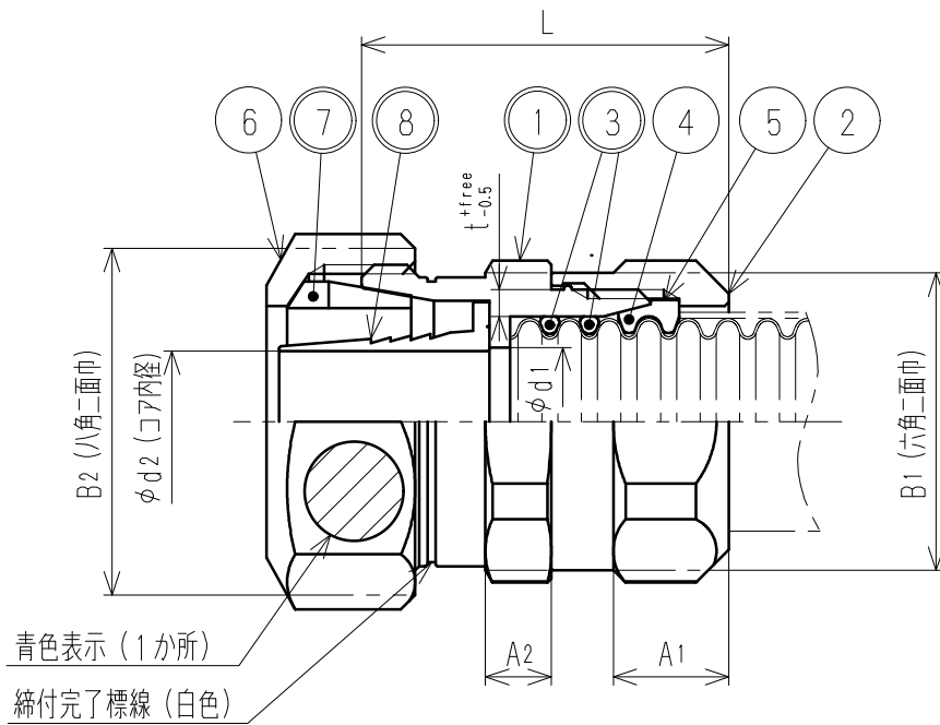
寸法表
