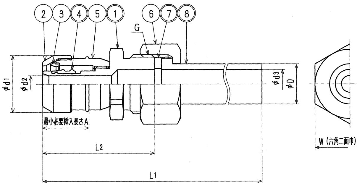
寸法表
