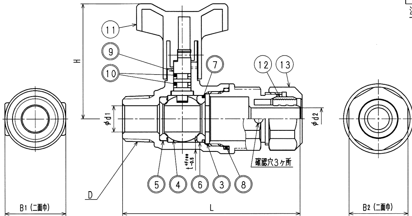
寸法表
