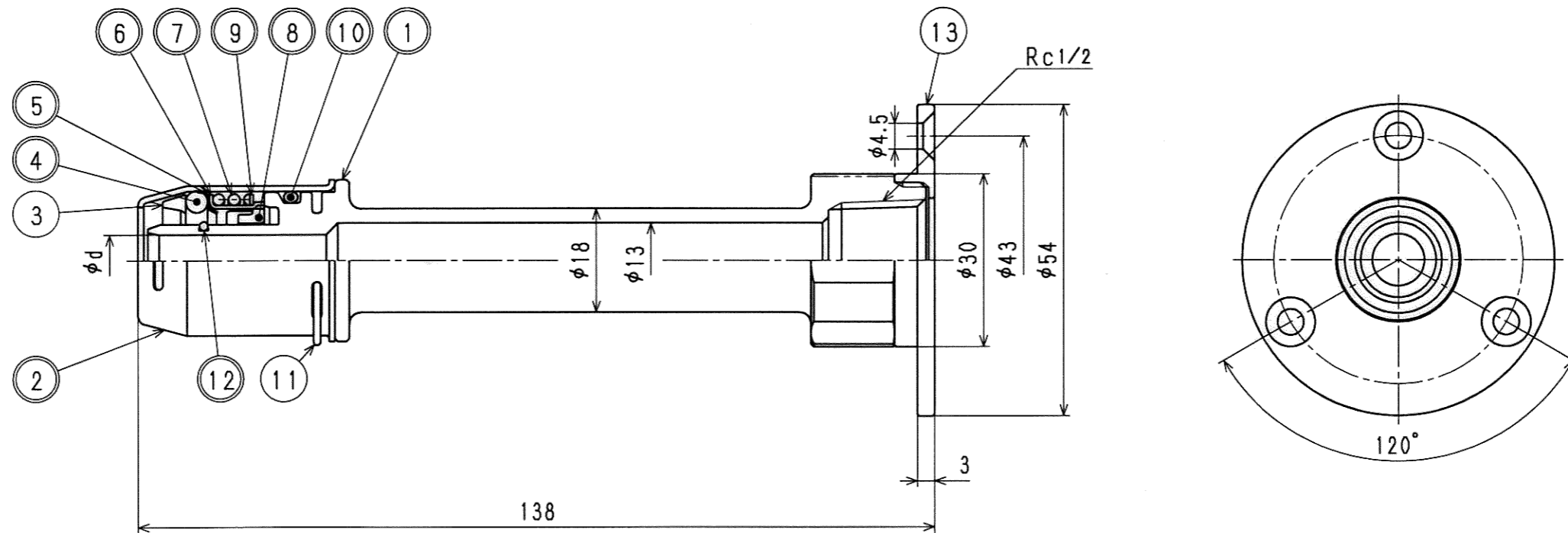
寸法表 (mm)
