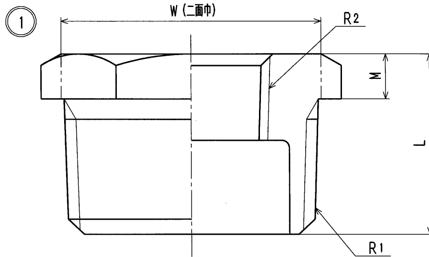
寸法表 (mm)
