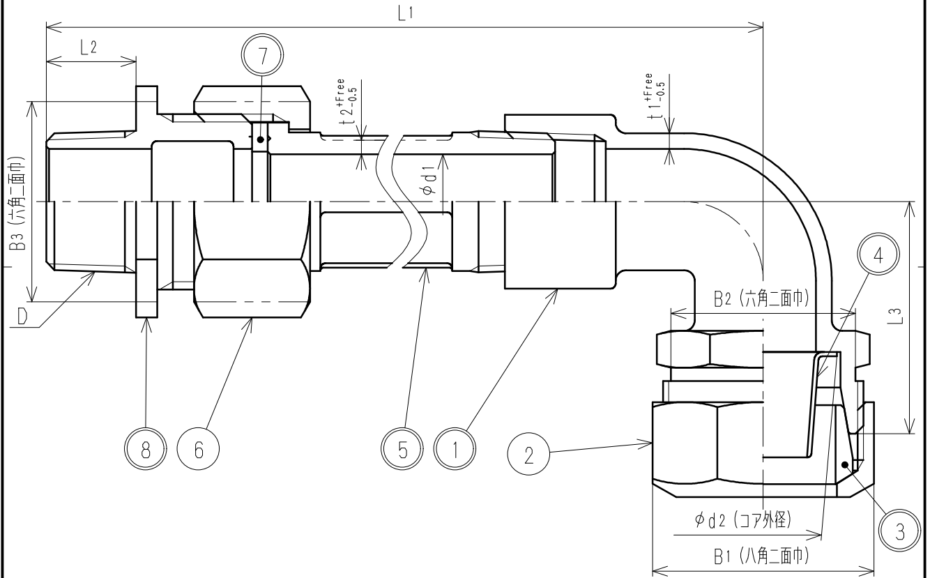
寸法表
