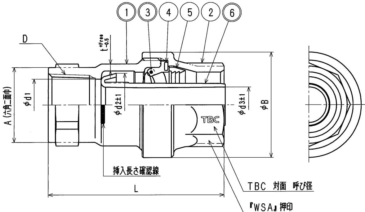
寸法表
