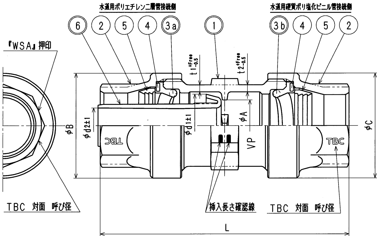
寸法表
