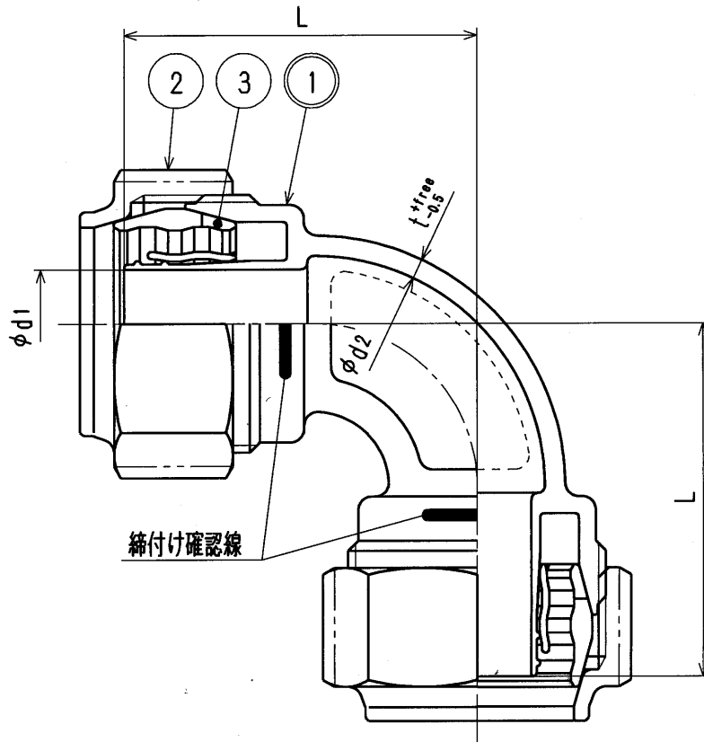
寸法表
