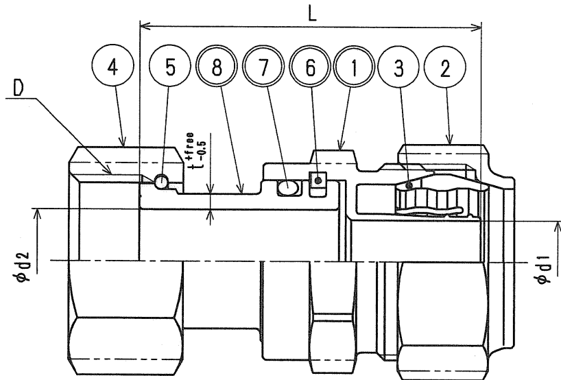
寸法表
