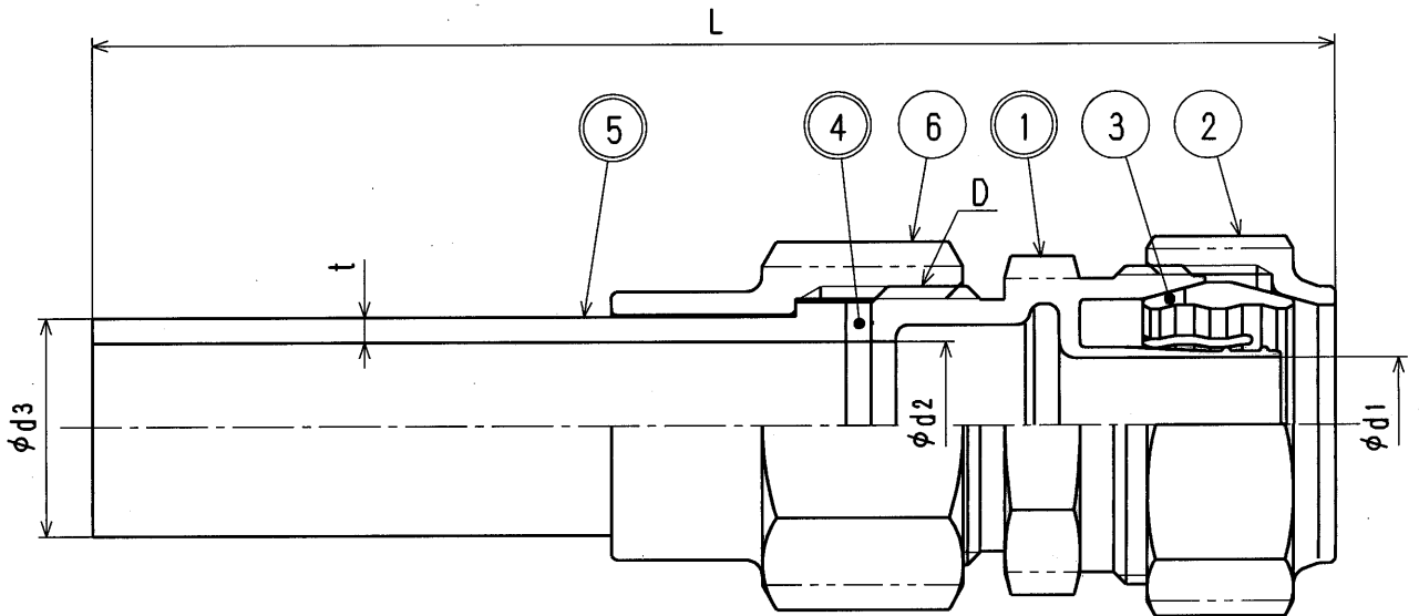
寸法表
