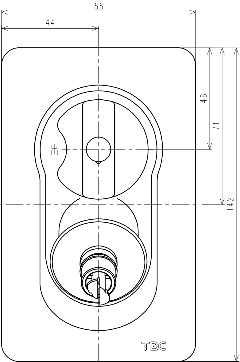
ハンドル（開）
