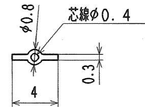
ビニタイ断面図
