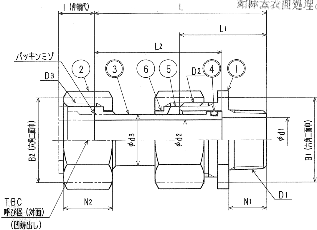
寸法表
