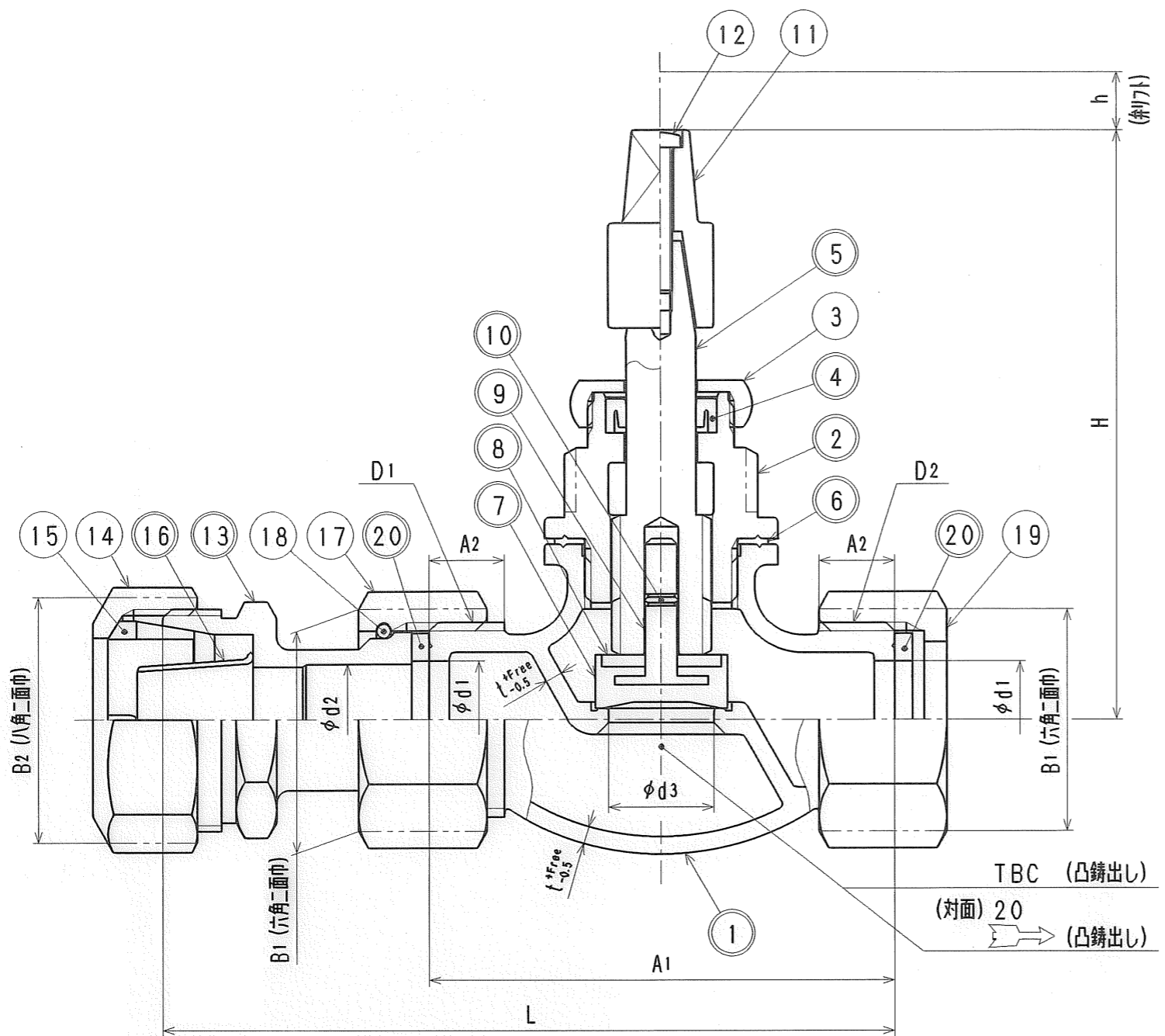
寸法表
