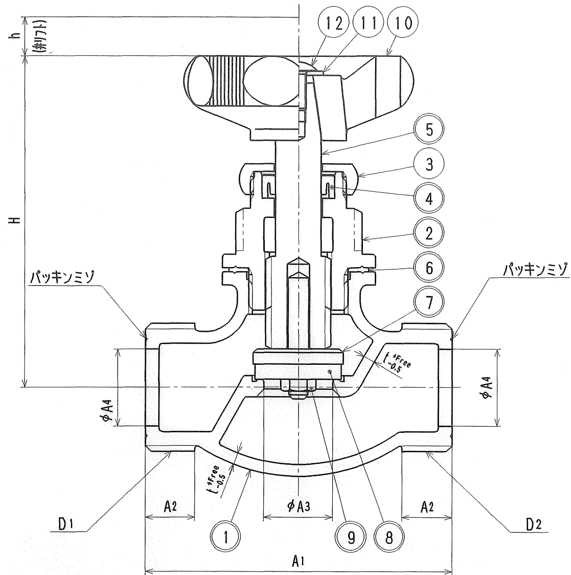
寸法表
