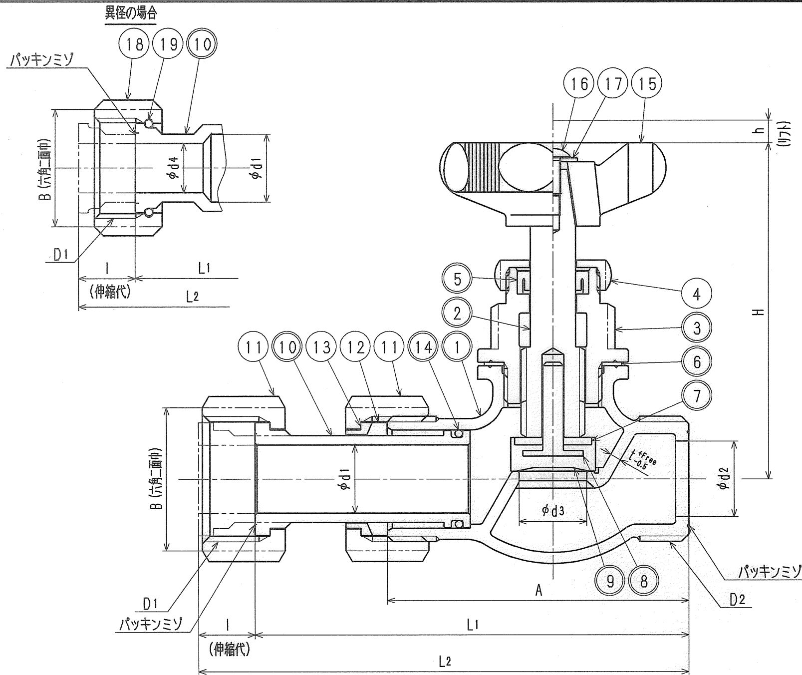
寸法表
