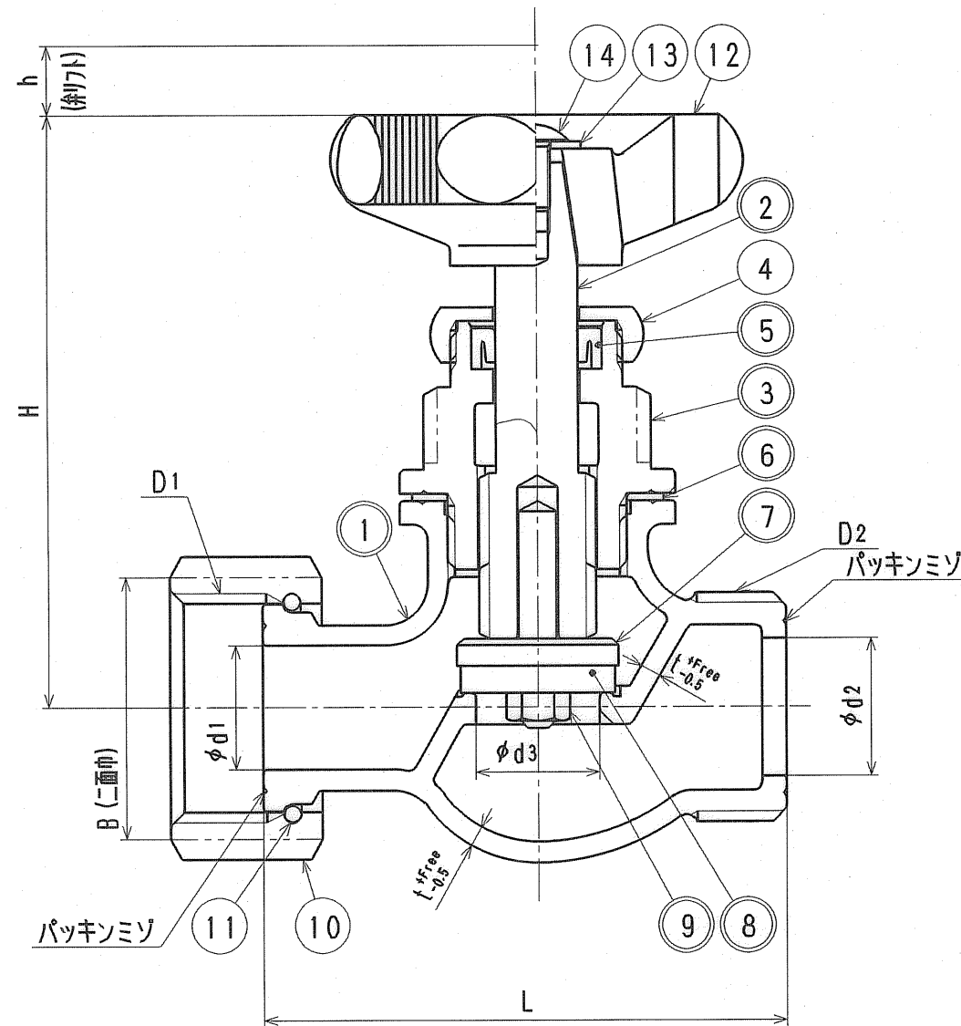
寸法表
